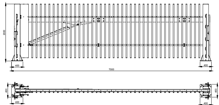
Beispiel Industrietor
